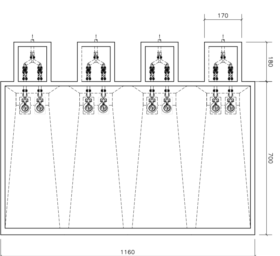
PLANIMETRIA TORRE DI POMPAGGIO
